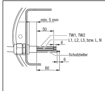
Рисунок 5: Вентилятор, встроенный в положении лёжа (Вал вертикально, ротор вниз), Прокладка кабеля в виде "водяного мешка"
